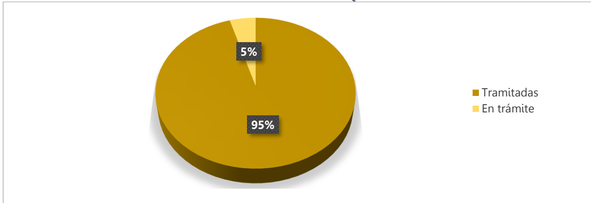
ILUSTRACIÓN 1: GESTIÓN PQRS
